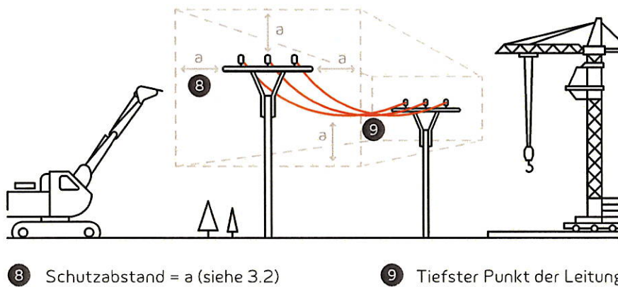
Abb. 5: Schutzabstände am Beispiel einer Freileitung mit einer Spannung von 20.000 Volt, ohne Windeinfluss
