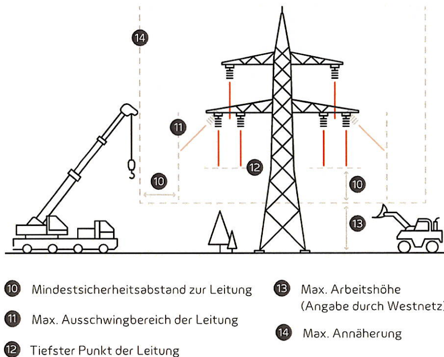
Abb. 6: Schutzabstände am Beispiel einer Freileitung mit einer Spannung von 110.000 Volt, mit und ohne Windeinfluss (Ansicht in Leitungsrichtung)
