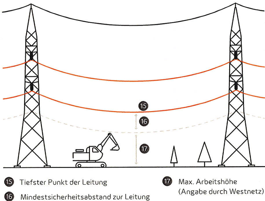
Abb. 7: Schutzabstände am Beispiel einer Freileitung mit einer Spannung von 110.000 Volt, mit und ohne Windeinfluss (Ansicht quer zur Leitungsrichtung)
