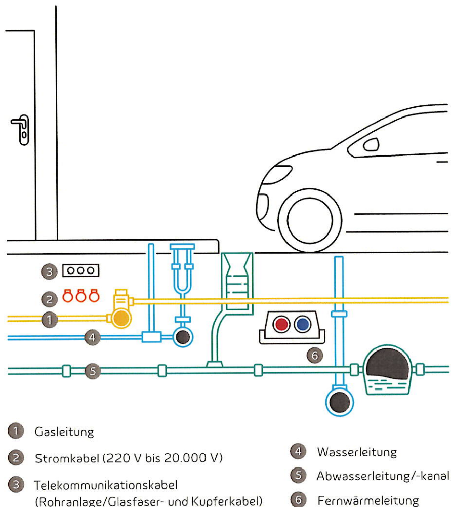
Abb. 1: Beispielhafte Lage von Versorgungsleitungen im Straßenzug
